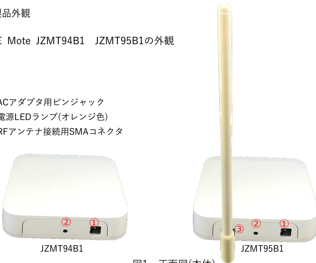
図1 正面図(本体)
